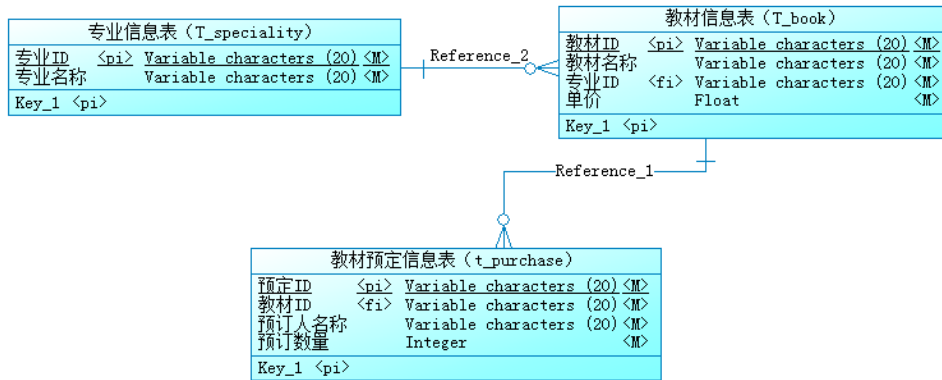
图 2.9.2 逻辑数据模型
