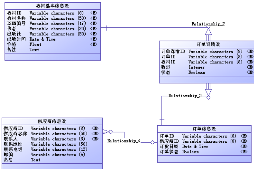
图 2.10.2 逻辑数据模型
