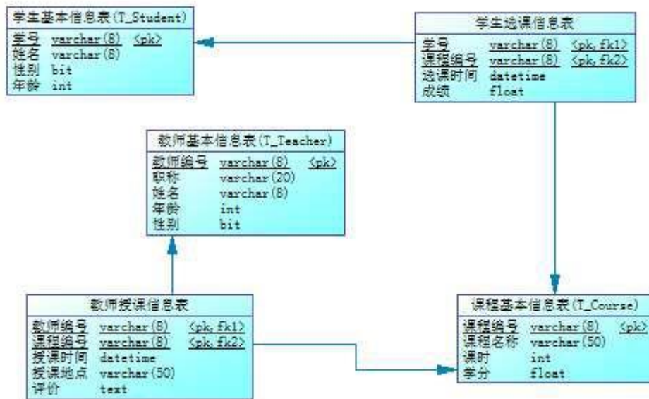
图 2.11.2 逻辑数据模型
