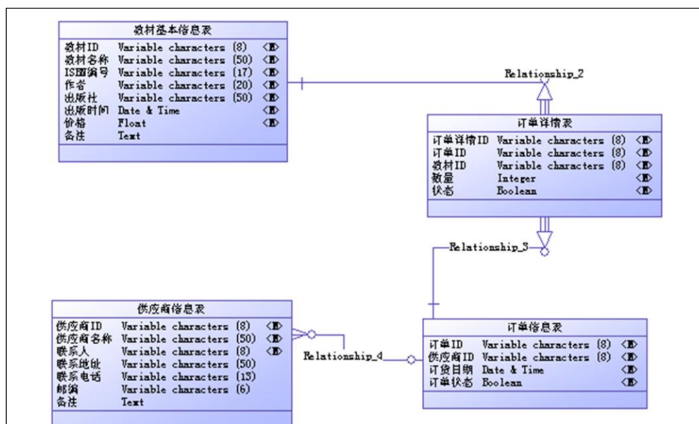
图 2.12.2 逻辑数据模型
