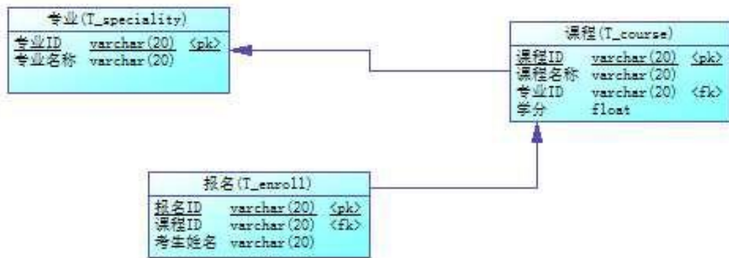
图 2.8.3 物理数据原型
