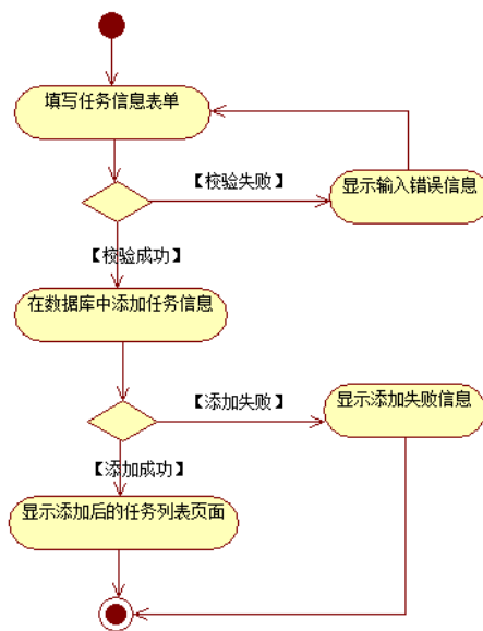
图 1.14.6 任务添加功能活动图
