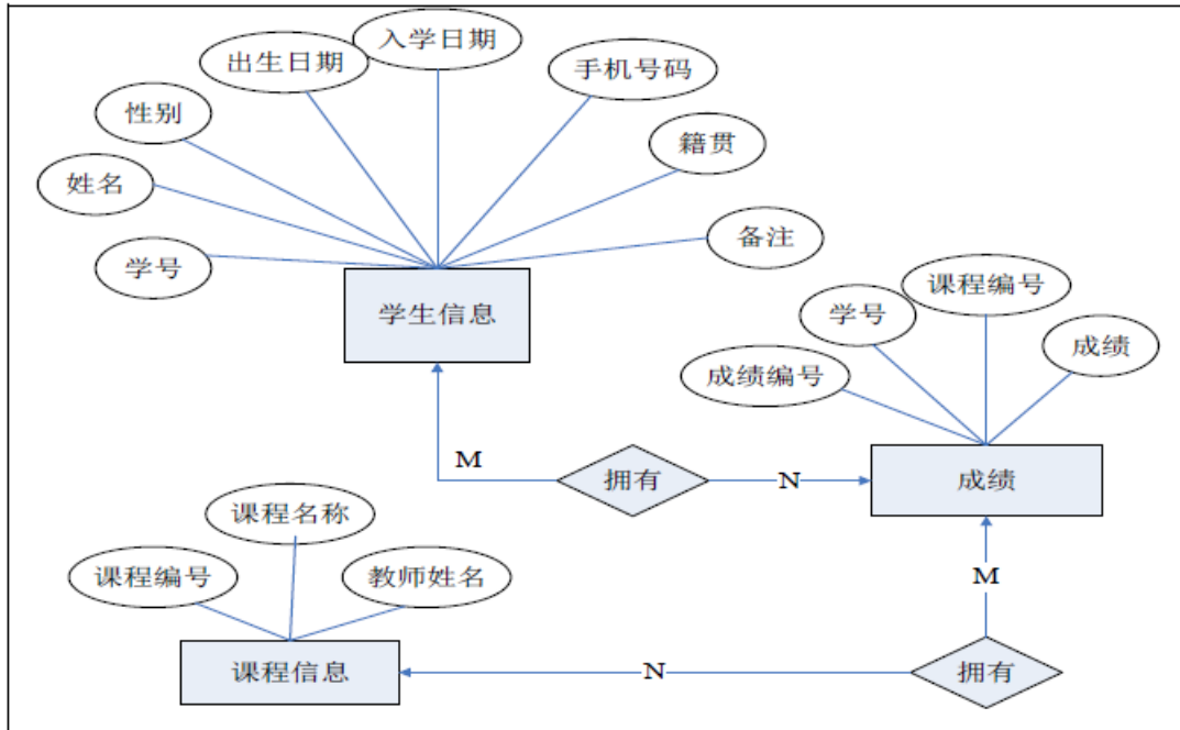
图 2.6.1 E-R 图
