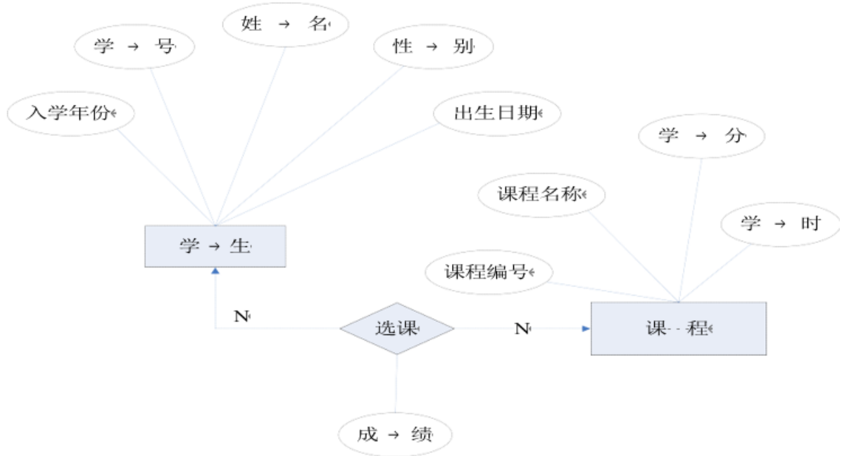
图 2.4.1 E-R 图
