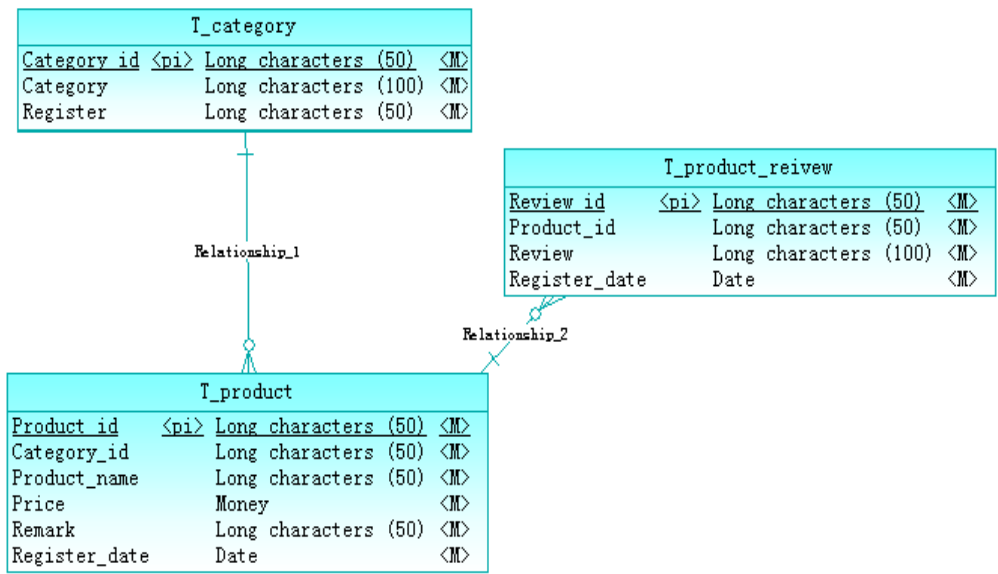
图 2.2.1 E-R 图
