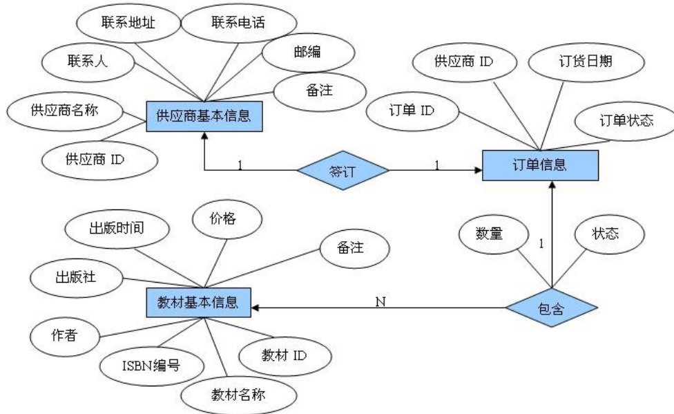
图 2.10.1 E-R 图
