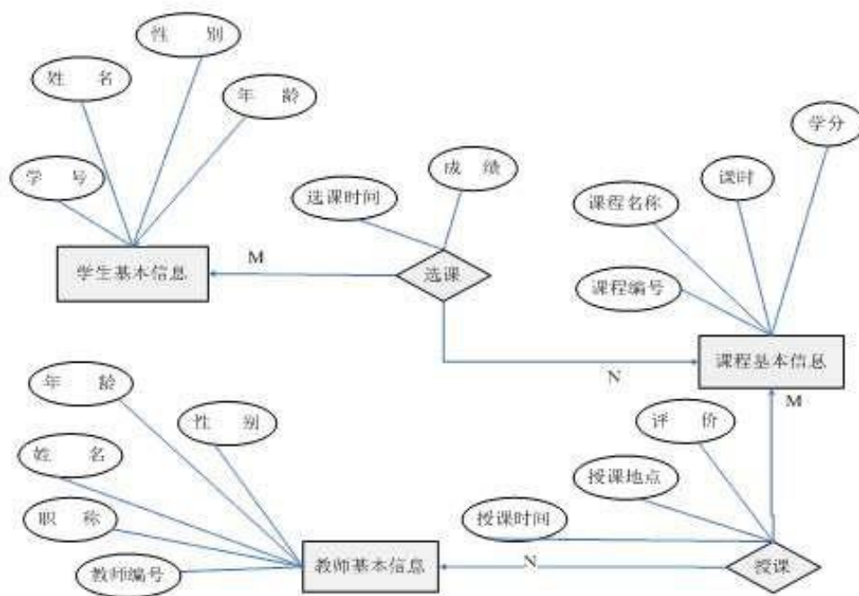
图 2.11.1E-R 图
