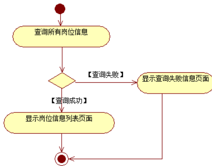
图 1.20.4 岗位信息列表显示活动图
