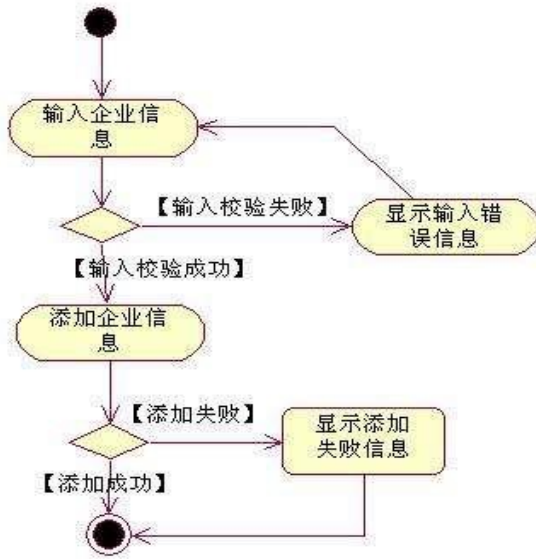
图 1.10.5 添加企业信息活动图
