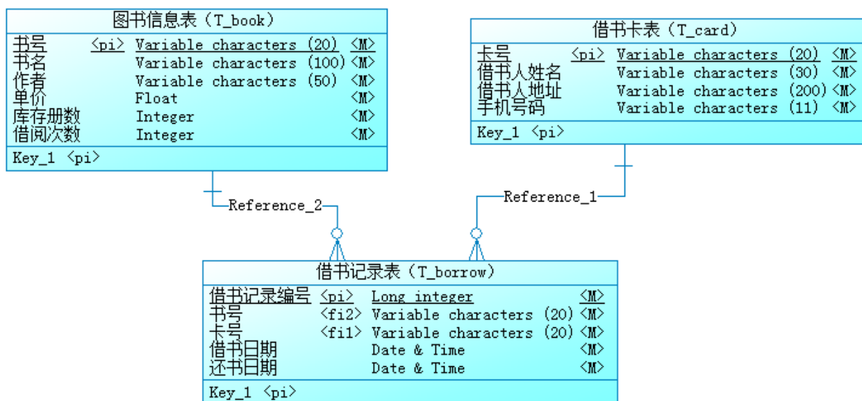
图 2.7.2 逻辑数据模型
