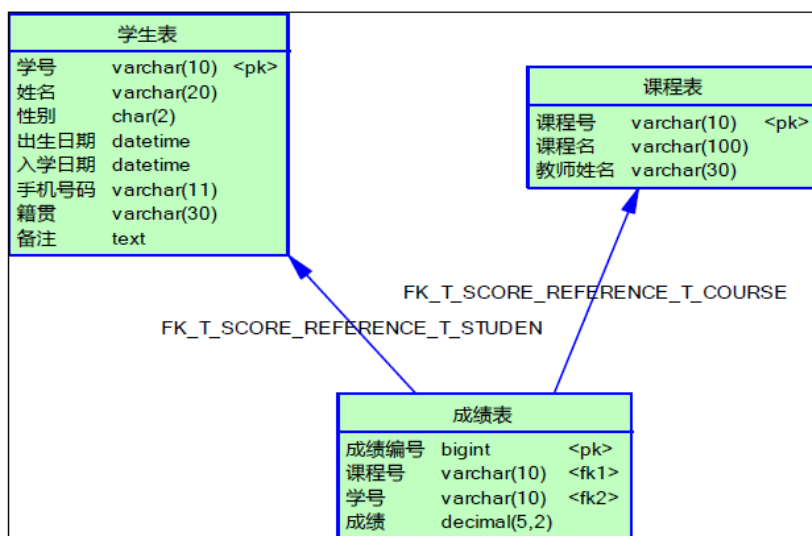
图 2.6.3 物理数据原型
