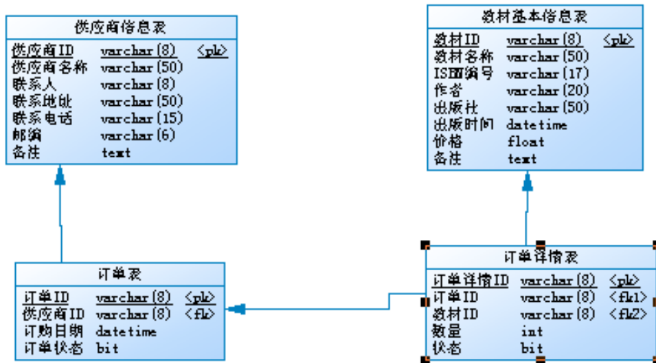
图 2.10.3 物理数据原型
