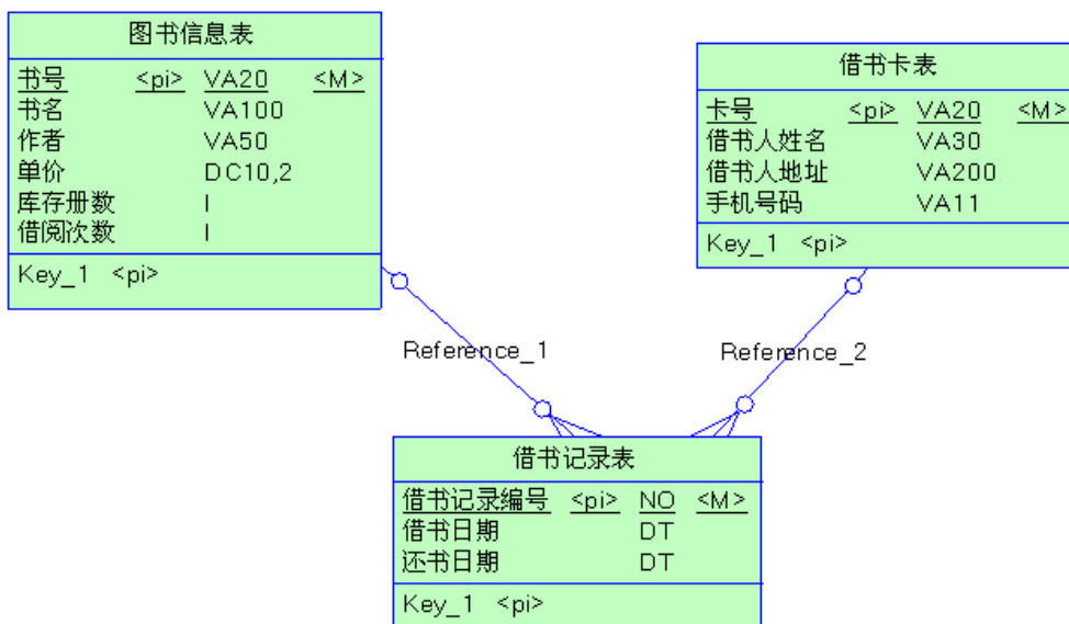
图 2.15.2 逻辑数据模型
