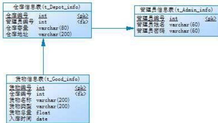
图 2.14.3 物理数据模型
