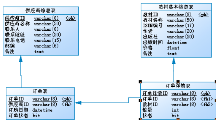
图 2.12.3 物理数据原型
