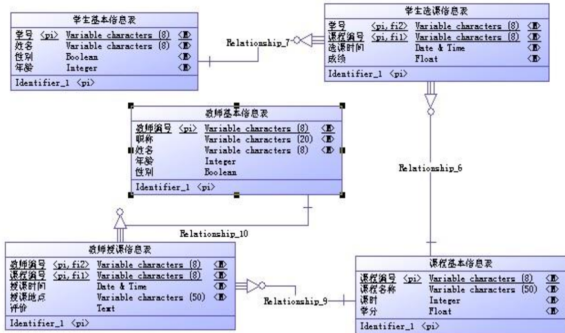
图 2.11.2 逻辑数据模型
