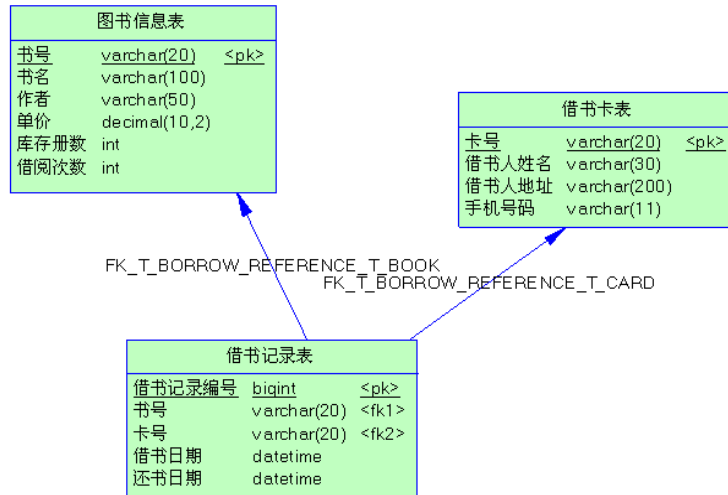
图 2.15.3 物理数据原型
