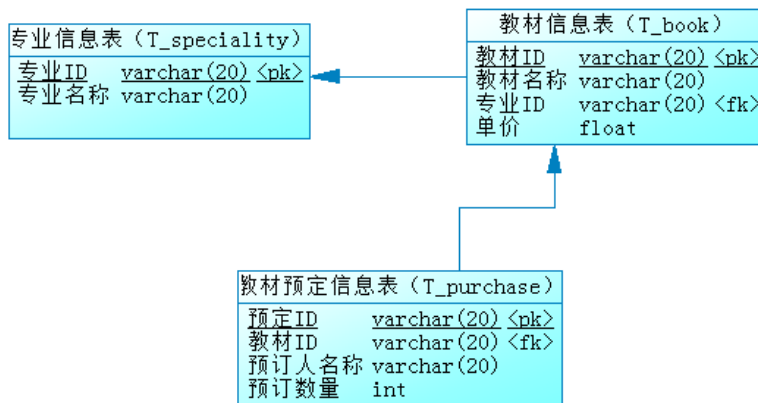
图 2.9.3 物理数据原型
