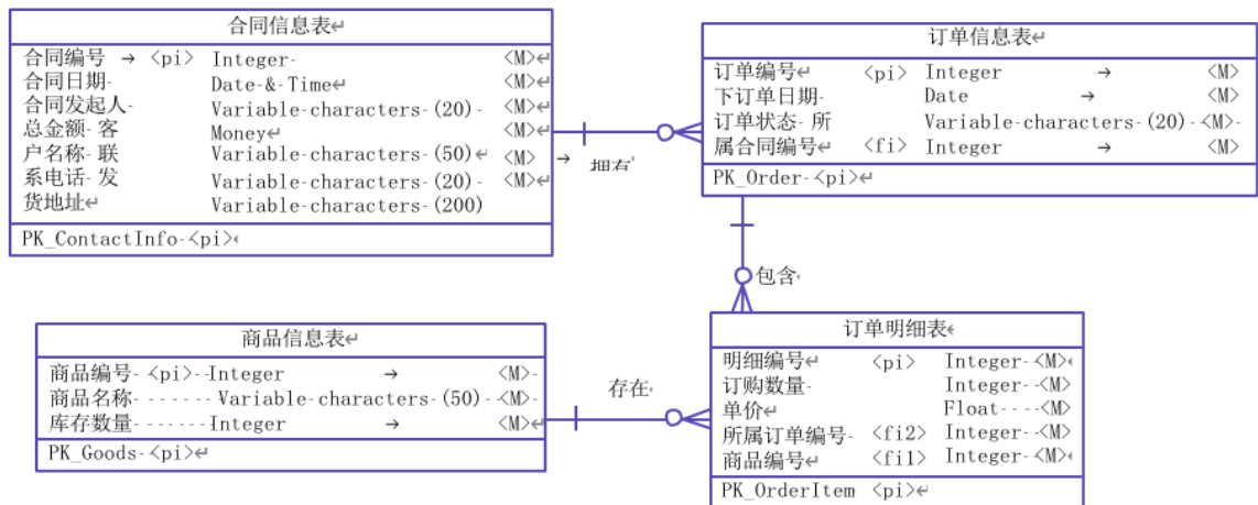
图 2.13.2 逻辑数据模型
