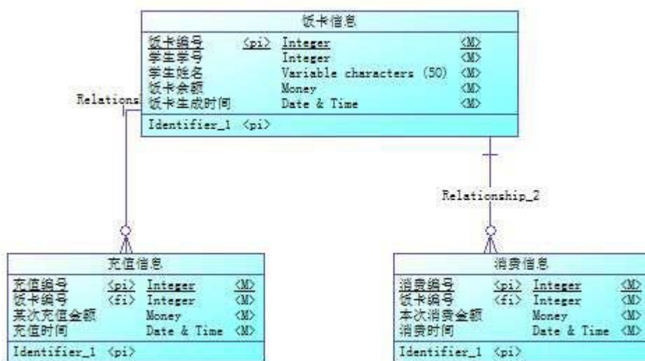
图 2.3.2 逻辑数据模型图
