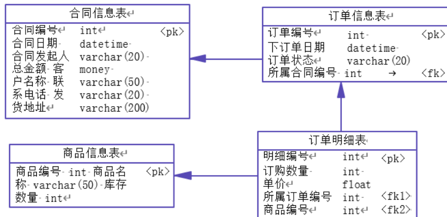
图 2.13.3 物理数据原型
