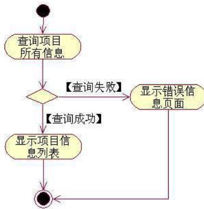
图 1.9.4 项目信息列表活动图
