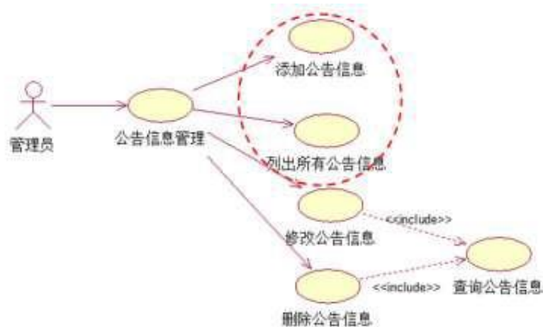
图 1.6.3 公告信息管理用例图
