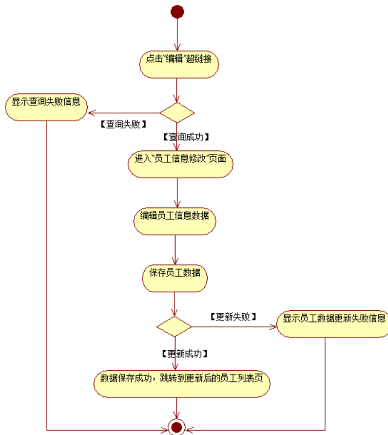
图 1.16.5 员工信息编辑功能活动图
