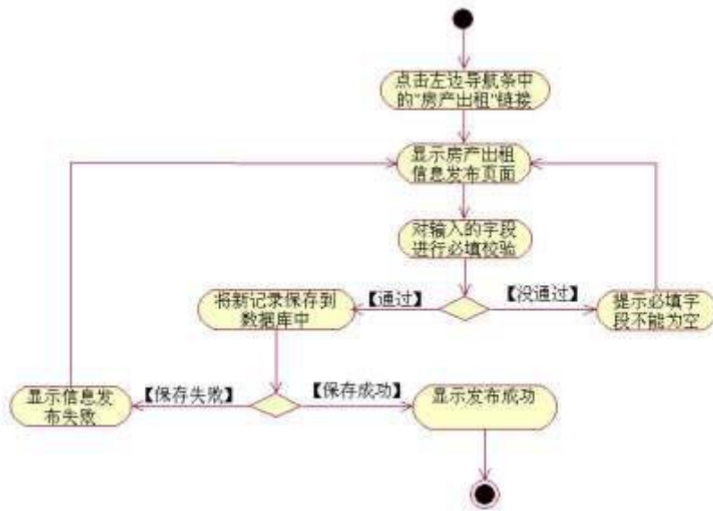
图 1.8.4 出租信息发布活动图
