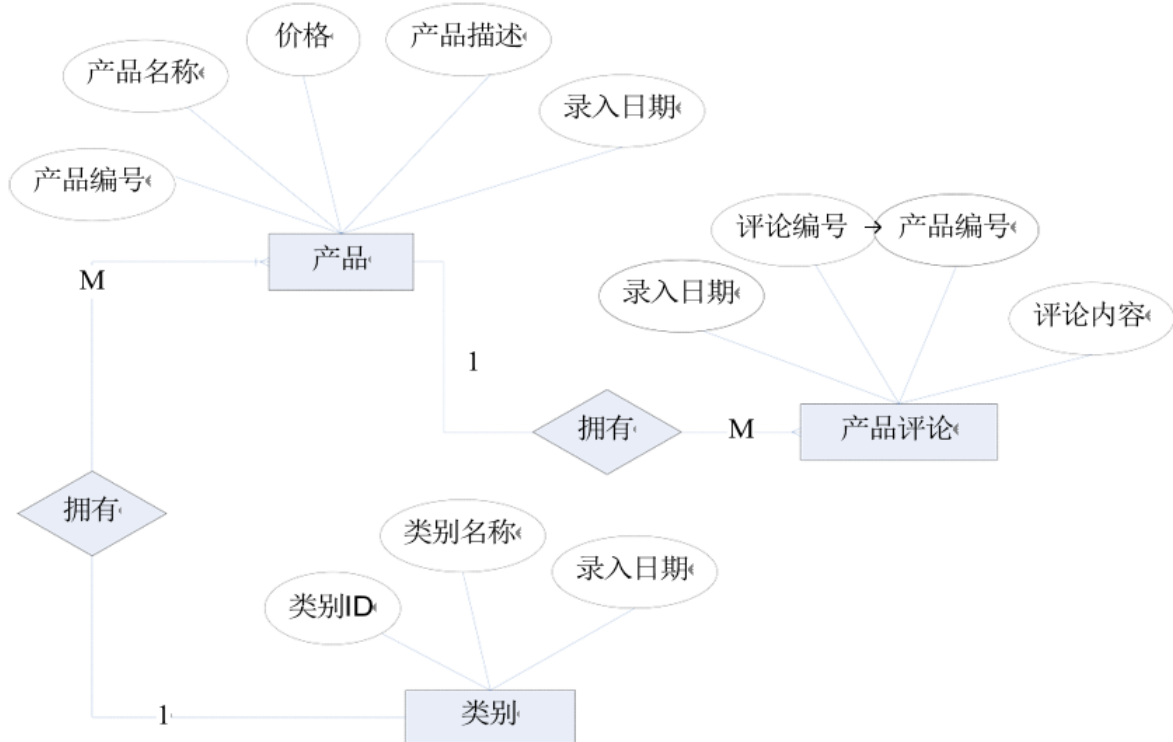
图 2.2.1 E-R 图
