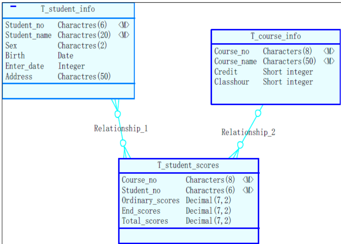
图 2.5.1 E-R 图
