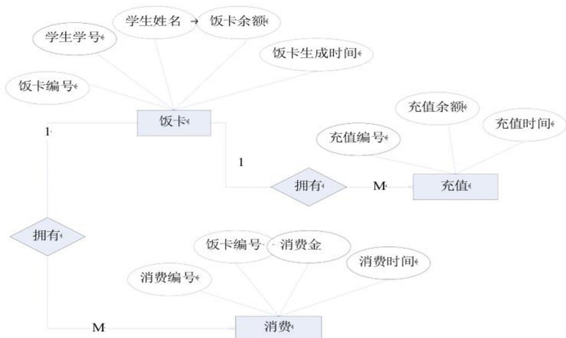
图 2.3.1 E-R 图
