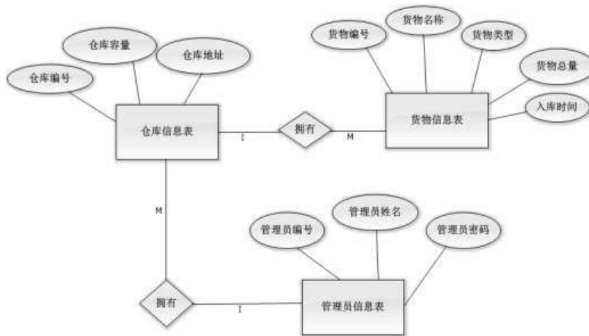
图 2.14.1 E-R 图
