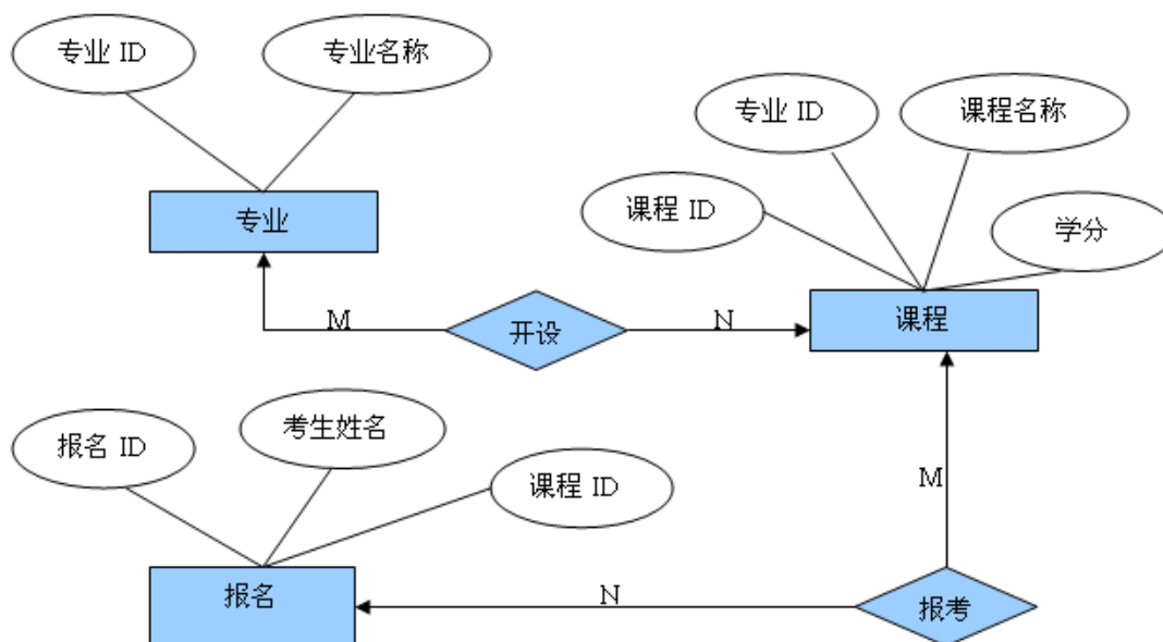
图 2.8.1 E-R 图
