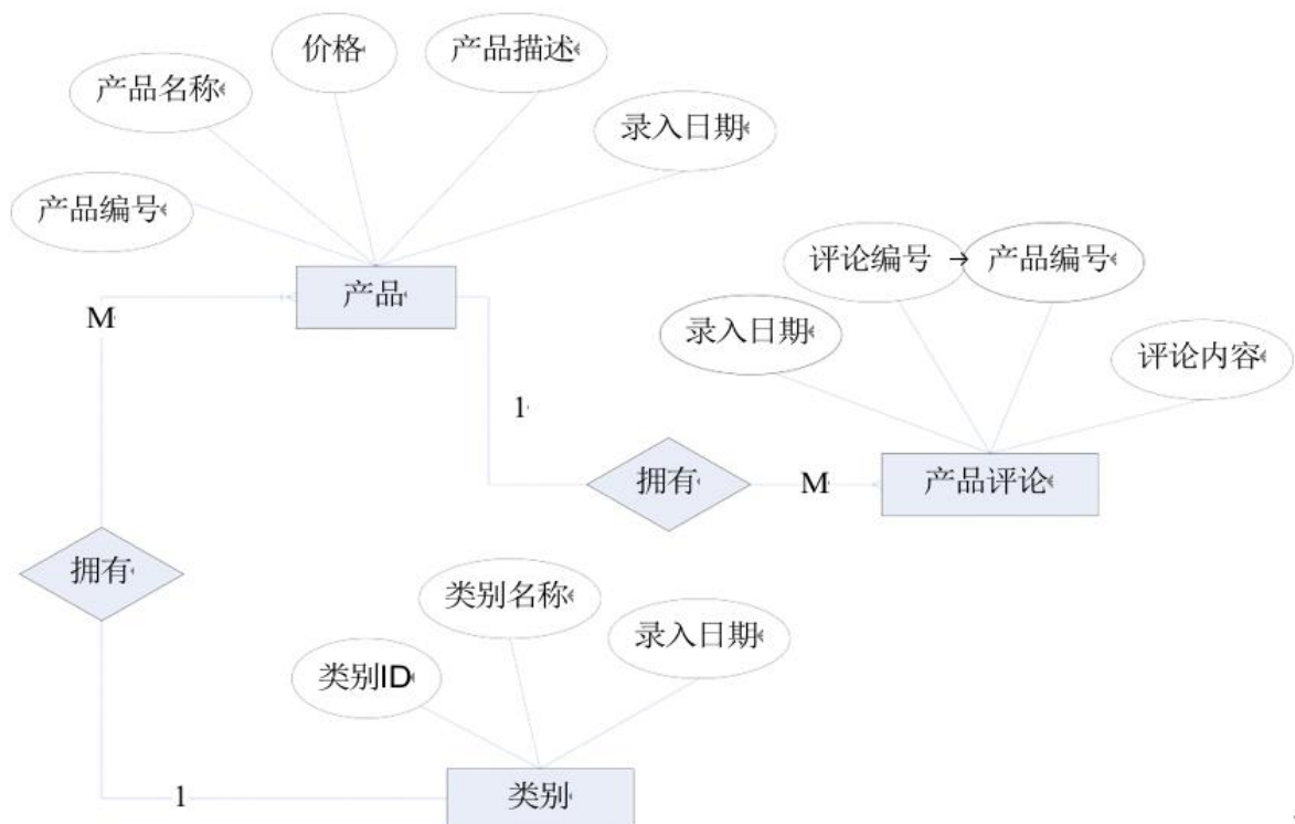
图 2.1.1 E-R 图
