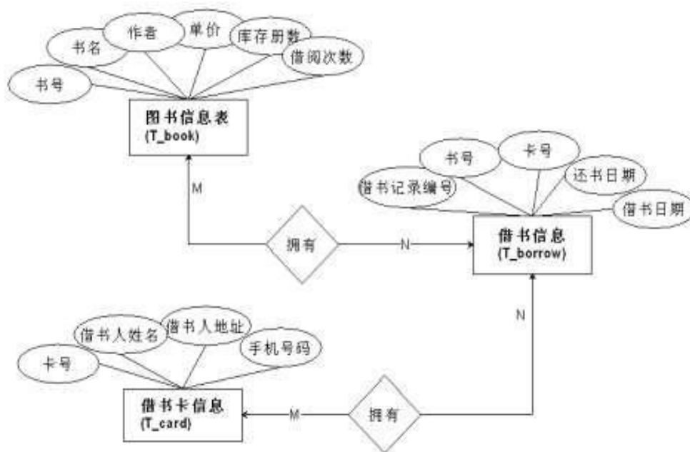
图 2.15.1 E-R 图
