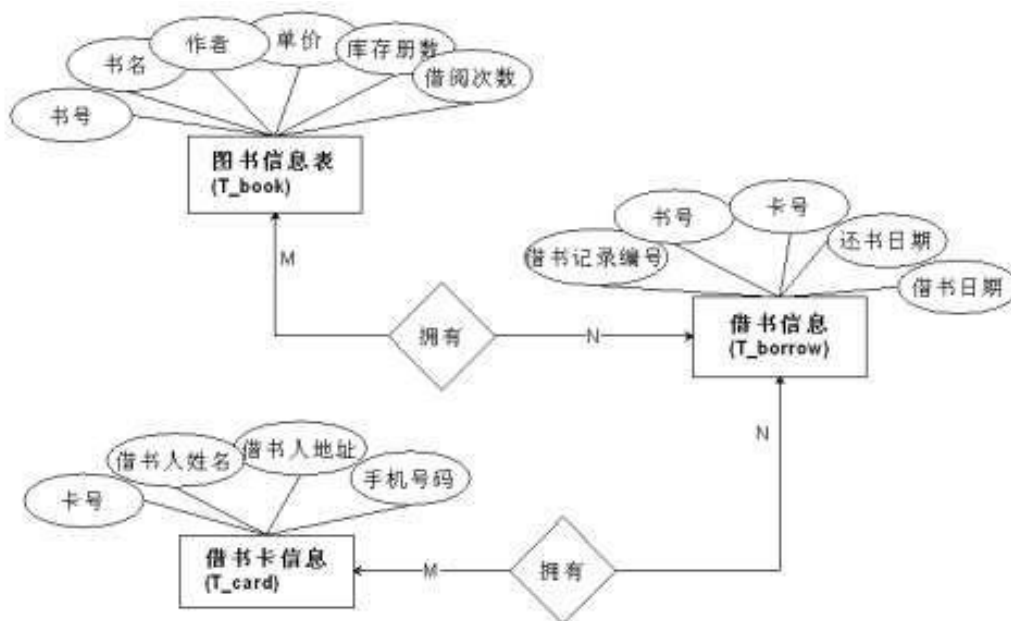
图 2.7.1 E-R 图
