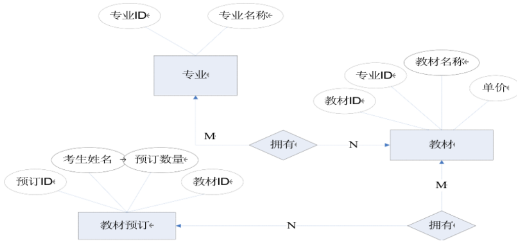
图 2.9.1 E-R 图
