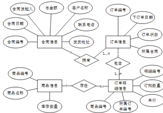
图 2.13.1 E-R 图
