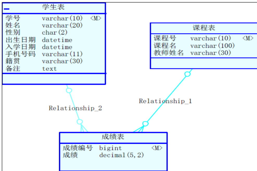
图 2.6.1 E-R 图
