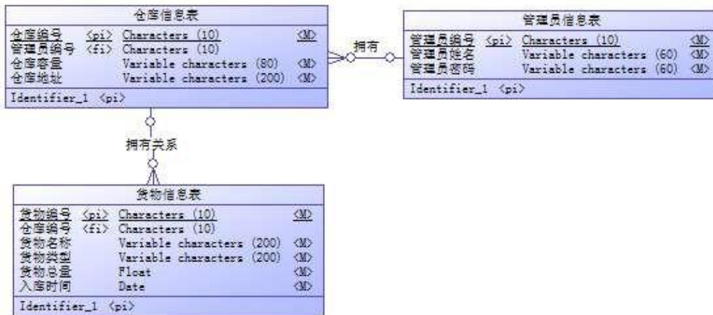
图 2.14.1 E-R 图
